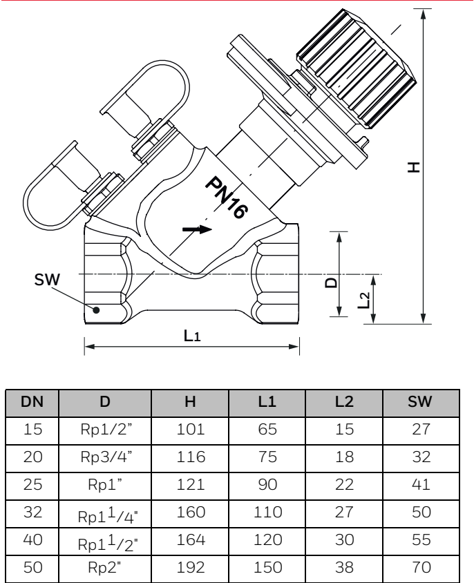
V5032...B Kombi-2-plus (DN15 - DN50)
