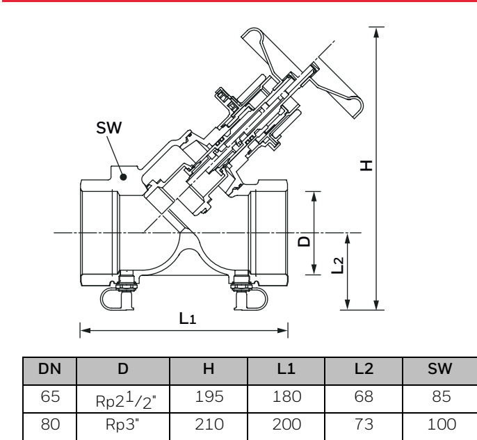
V5032...B Kombi-2-plus (DN65 - DN80)
